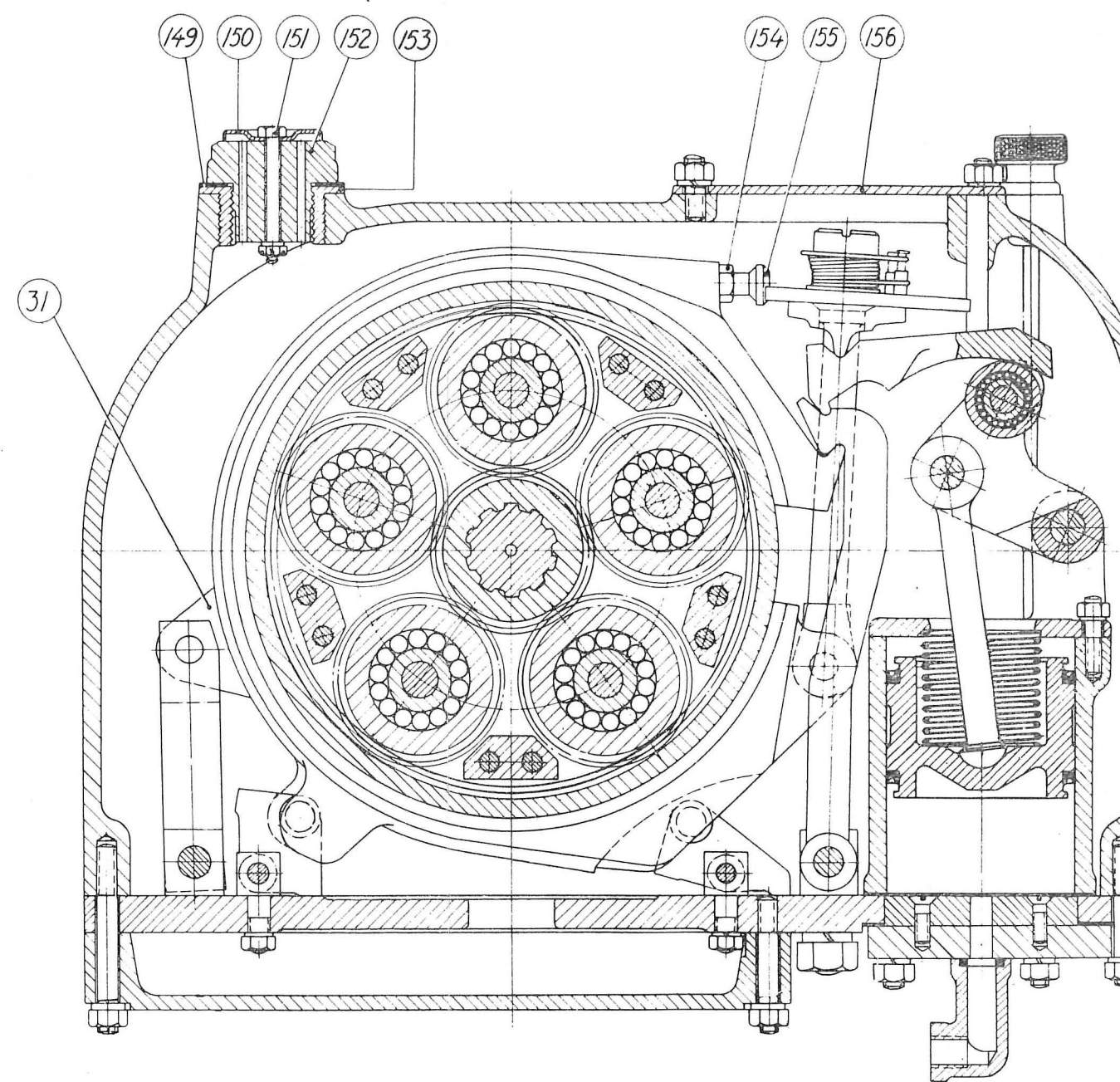
Växeln inkopplad
