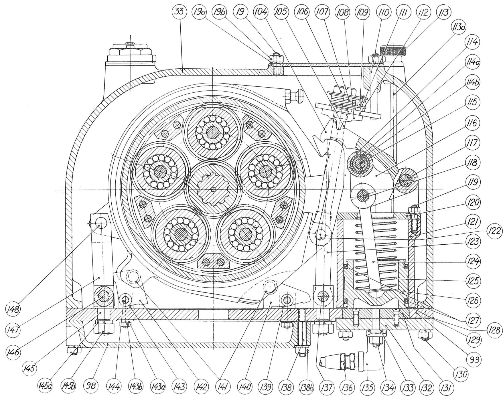
Växeln urkopplad
