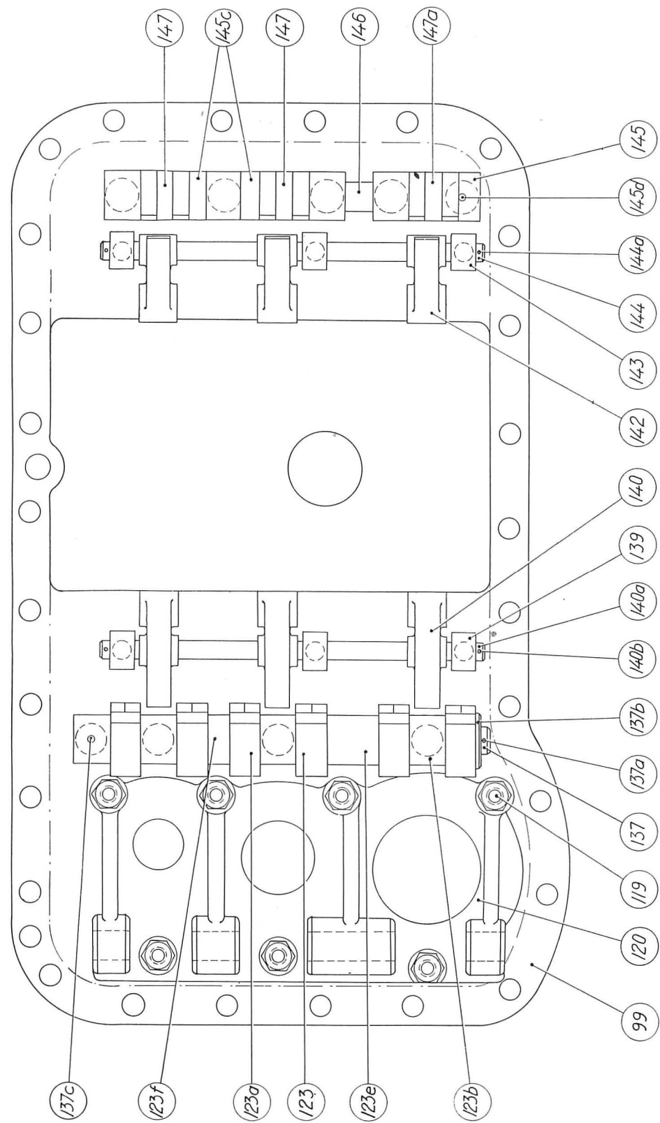
Bild 3 Bottenplatta
