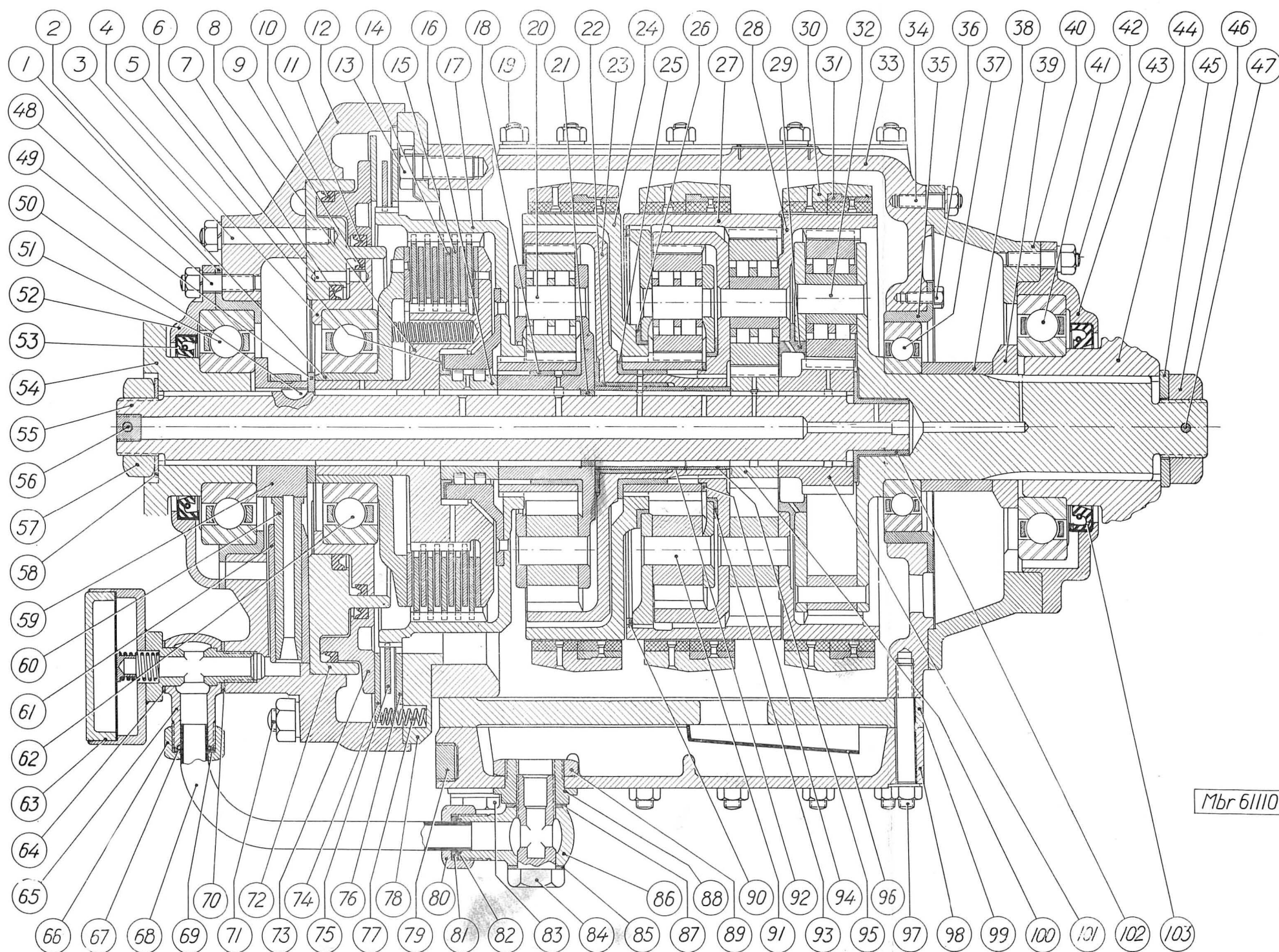
Bild 1 Wilsonväxel typ R11B. Längdsnitt
