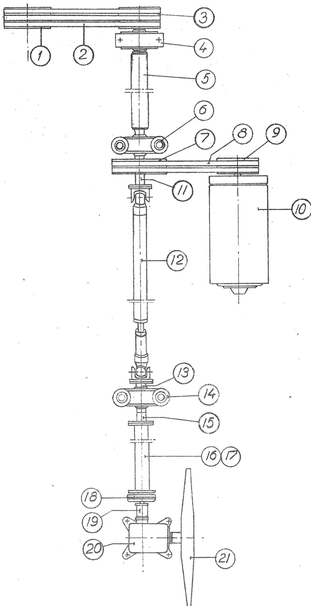
Fläkt-och generatordrivning
