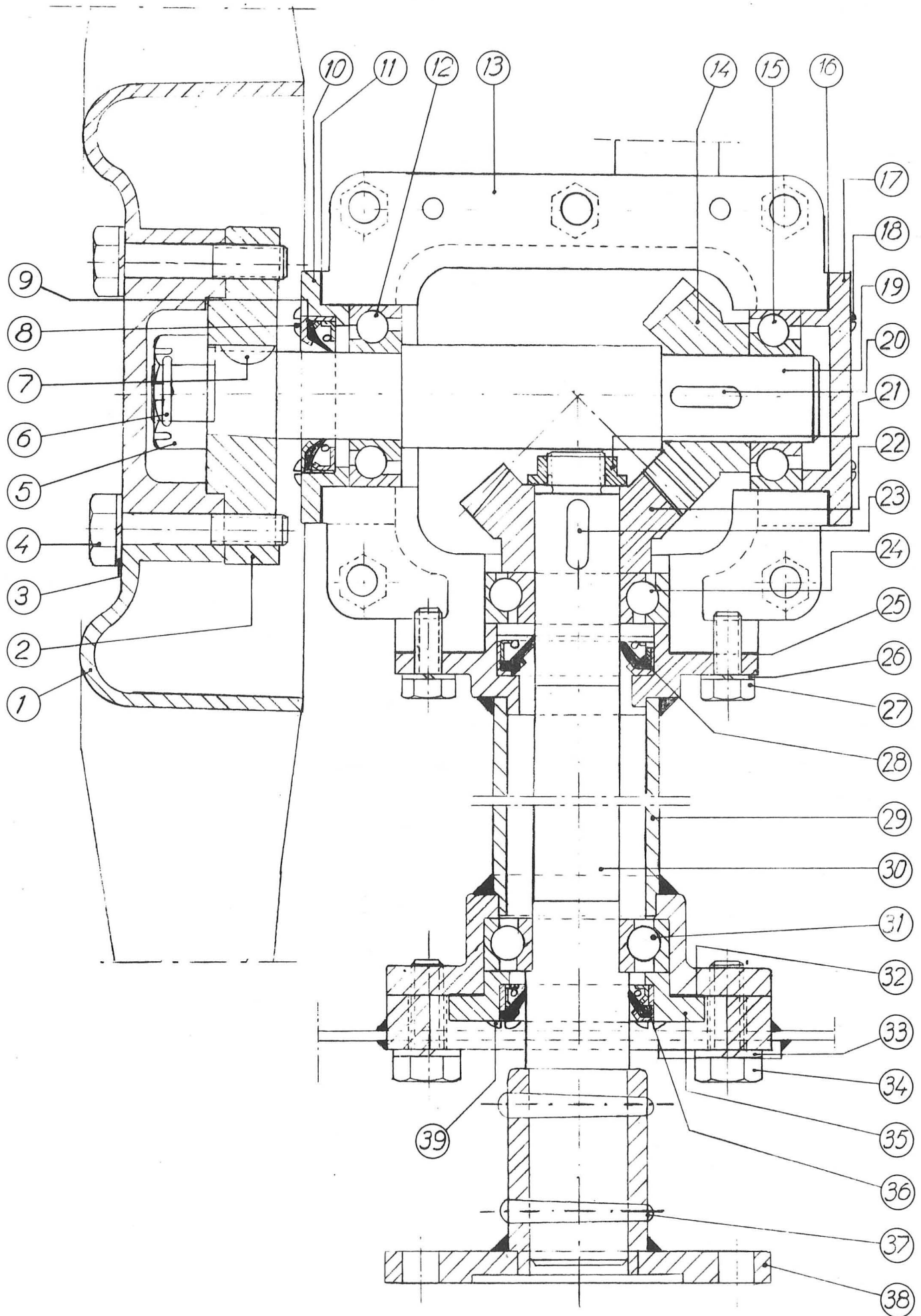
Kuggväxel. Fig. 7
