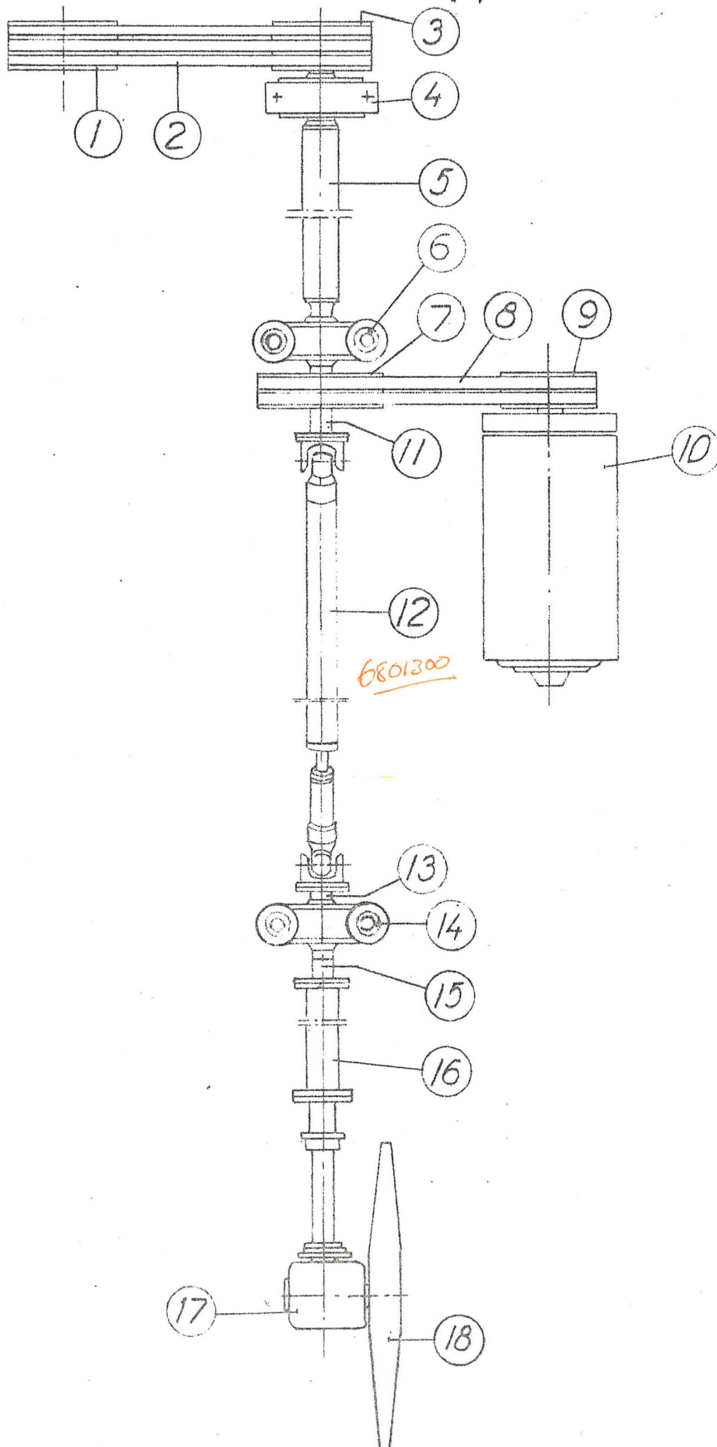
Fläkt- och generatordrivning Fig. 6.
