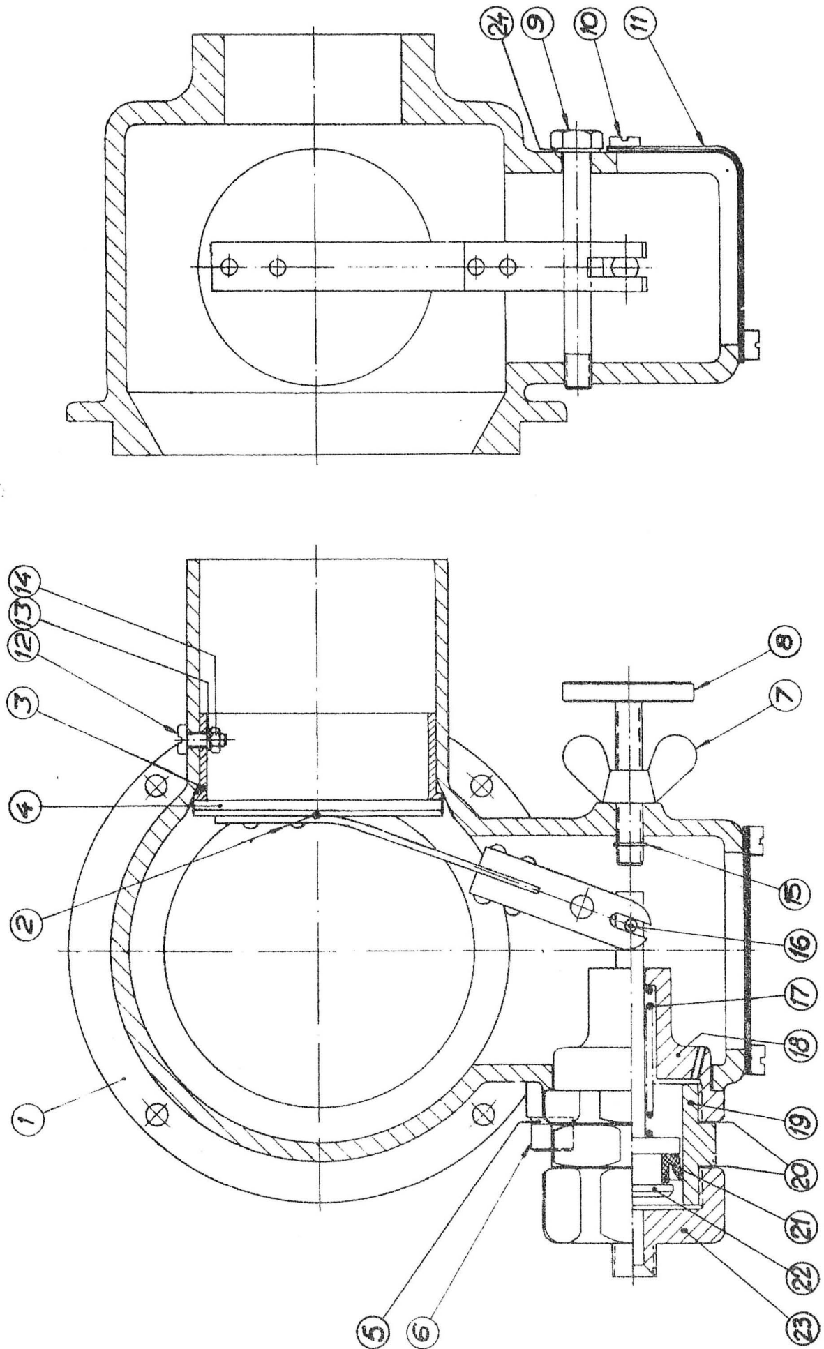
Luftintag med backspjäll Fig. 2.
