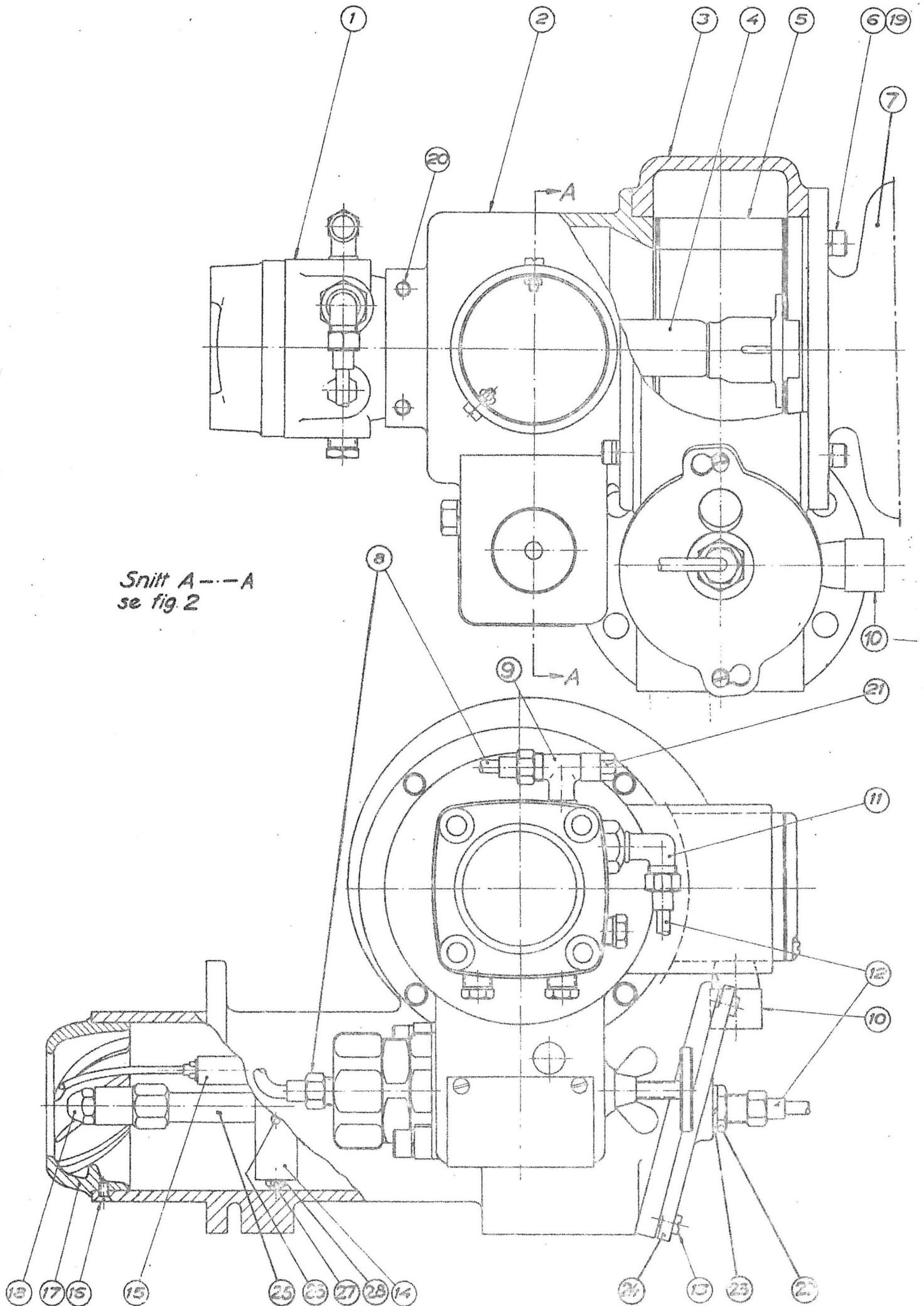
Oljebrännare HT-35-RB/D Fig. 1
